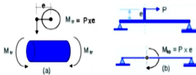
Gambar 2.16 (a) Momen puntir, (b) Momen Kopel
