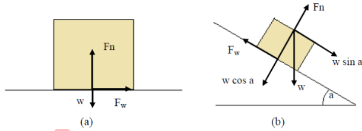
13 Gambar 2.21 Gaya gesek : (a) bidang datar ; (b) bidang miring
