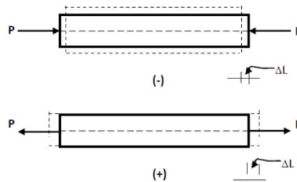
Gambar 2.22 Pengaruh Gaya Normal Pada Balok
