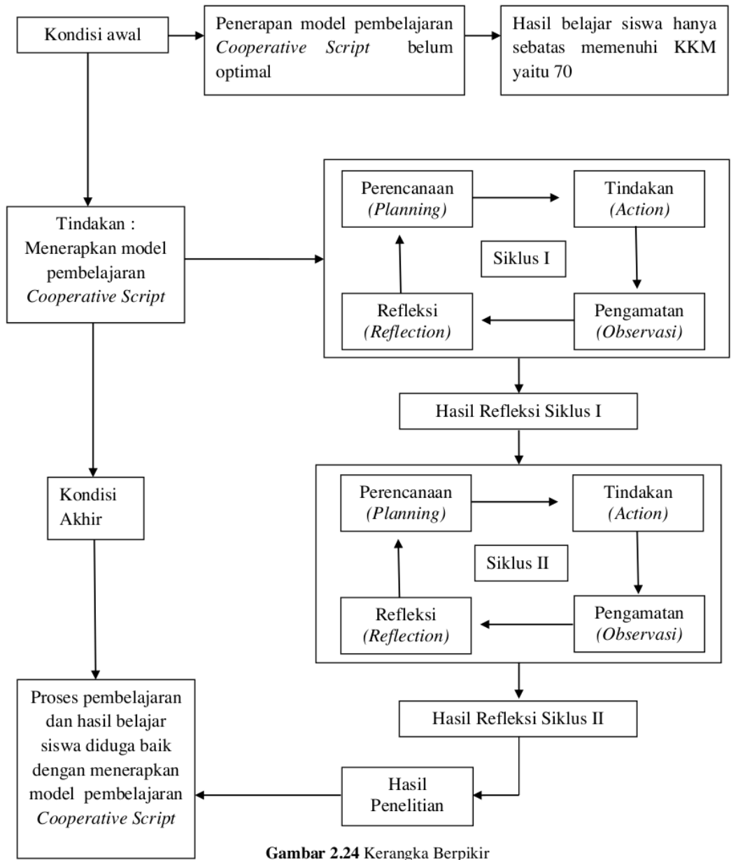
Gambar 2.24 Kerangka Berpikir
