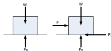
Gambar 2.20 Gaya Gesek
