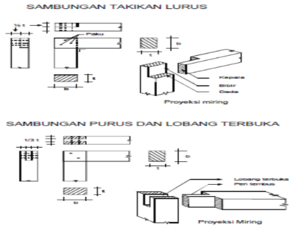
Gambar 10 : Samb. Takikan Lurus Dan Lobang Terbuka. (Sumber :Bahan ajar konstruksi bangunan jilid 2)
