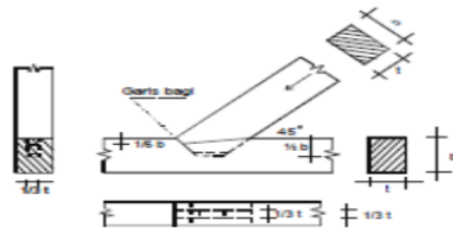
Gambar 14 : Samb. Purus Dan Lobang Dengan Gigi Tegak Dan Purus Lobang Dengan Gigi Garis Bagi.
