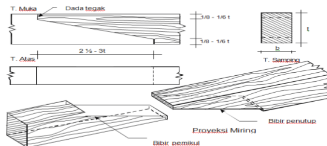
Gambar 8 : Sambungan Bibir Miring
