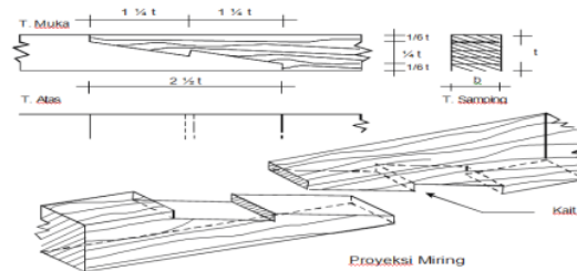
Gambar 9 : Sambungan Bibir Miring Berkait (Sumber :Bahan ajar konstruksi bangunan jilid 2)
