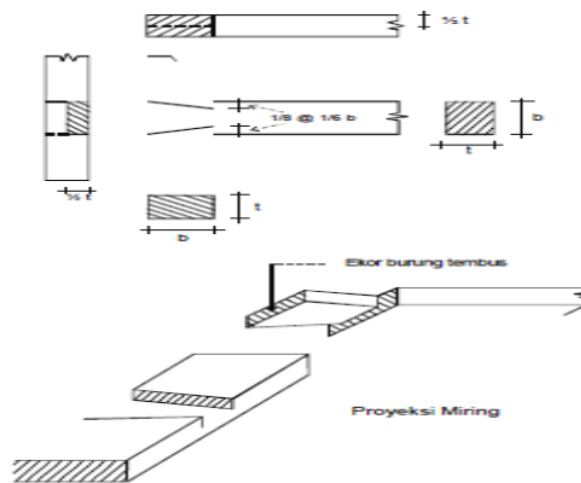
Gambar 12 : Sambungan Takikan Lurus Ekor Burung Pada Pertemuan.
