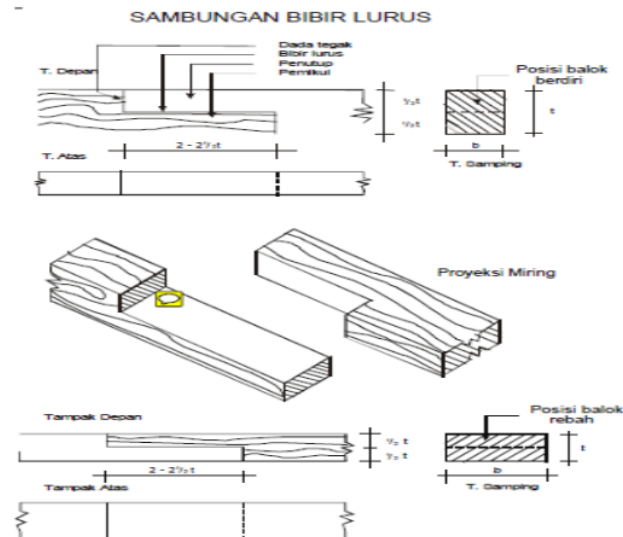
Gambar 6 : Sambungan Bibir Lurus
