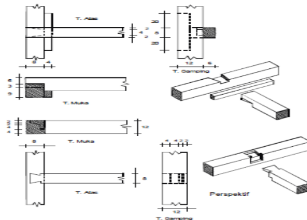
Gambar 15 : Samb. Takikan Lurus Ekor Burung Dengan Perkuatan Dan Samb Raveling Ekor Burung.
