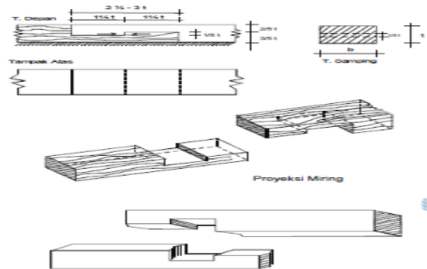
Gambar 7 : Sambungan Bibir Lurus Berkait
