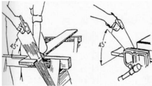
Gambar 4 : Memotong Kayu Secara Manual.
