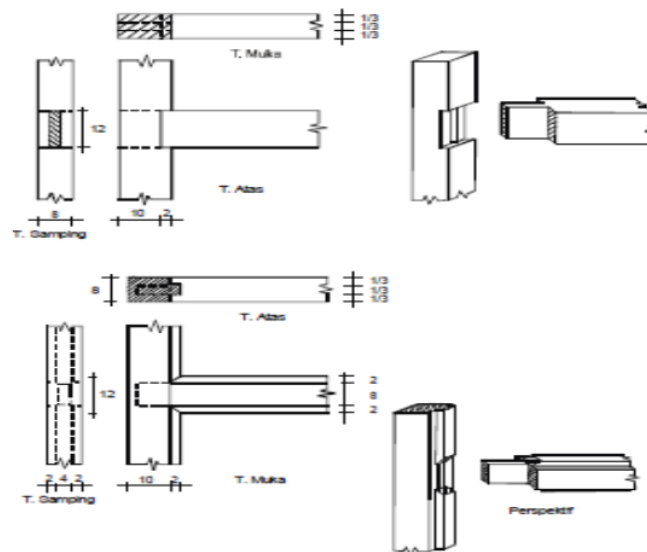
Gambar 13 : Samb. Purus Lobang Terbuka Dan Tertutup.
