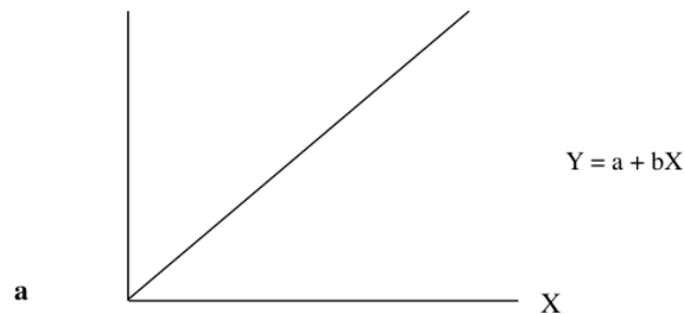
Gambar 3.2 Ilustrasi Garis Regresi Linear
