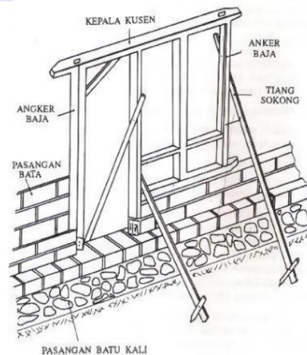
Gambar 2.8 Pemasangan Kusen Kayu
