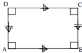
Gambar 2.8. Persegi Panjang ABCD
