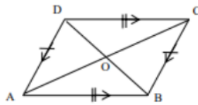
Gambar 2.7. Jajaran genjang ABCD
